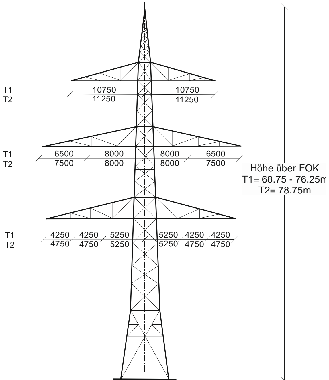
Schemazeichnung (ohne Maßstab) Maßangaben in Millimeter
